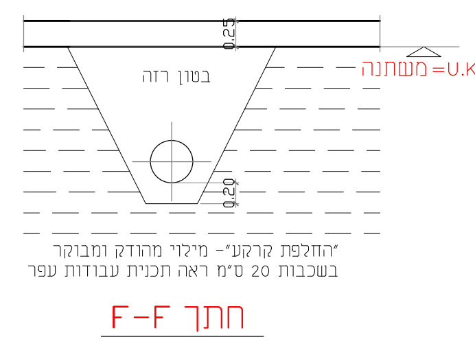
F-F תתך
