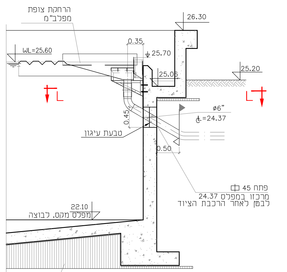
E-E חתך 1:50
