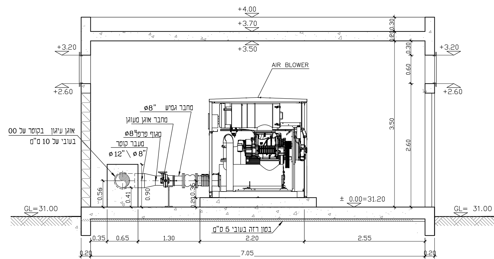
2-2 TTP
