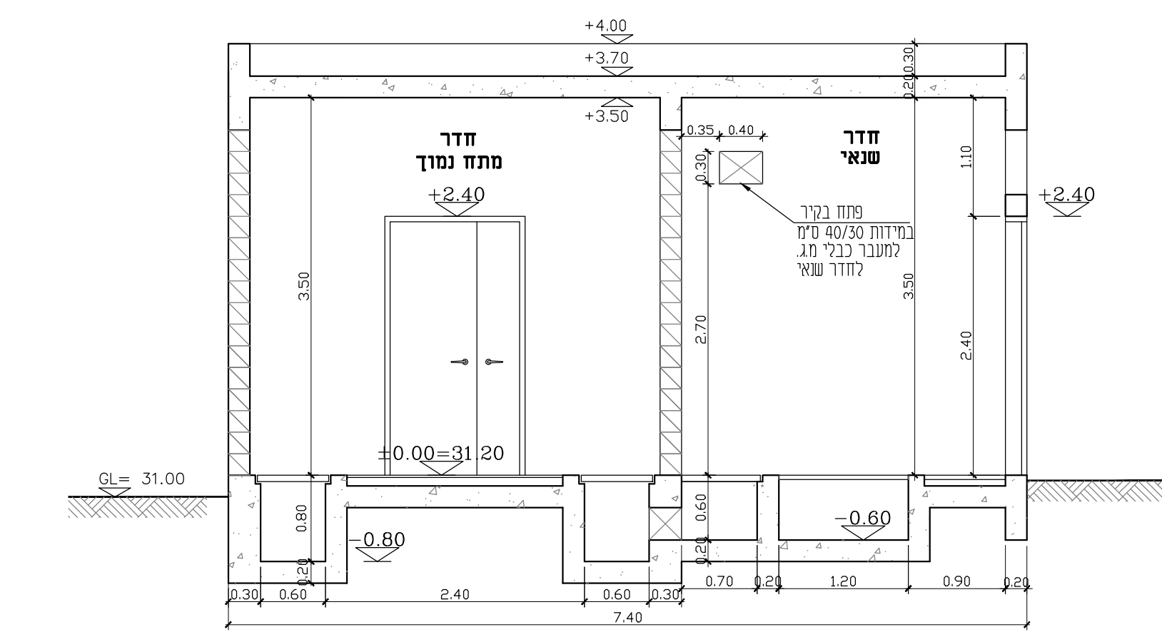
3-3 TTP
